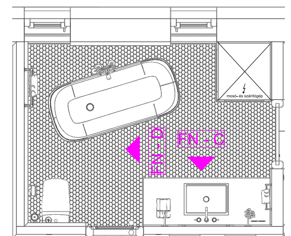
Alaprajz M= 1:50
