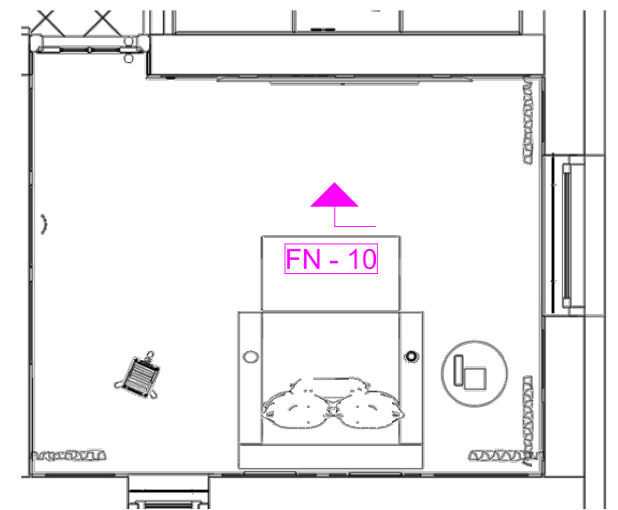
Alaprajz M= 1:50
